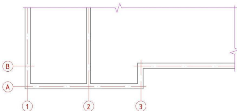
20P.10 pav. Mūrinio pastato ašių tinklėlis
